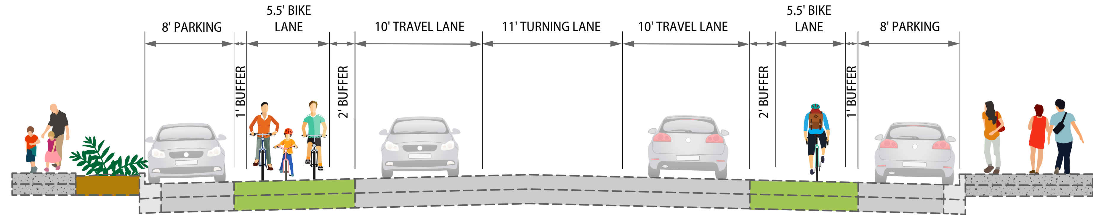
SECTION A-A
