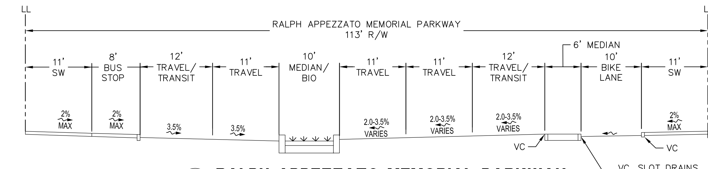
E RALPH APPEZZATO MEMORIAL PARKWAY NTS
