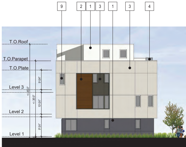
2.LEFT ELEVATION
